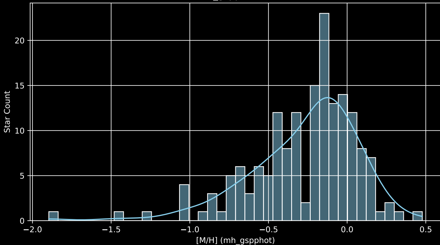
APOGEE DR17 Field: [283-23-O_TESS [M/H] (mh_gspphot) (n= 168)
