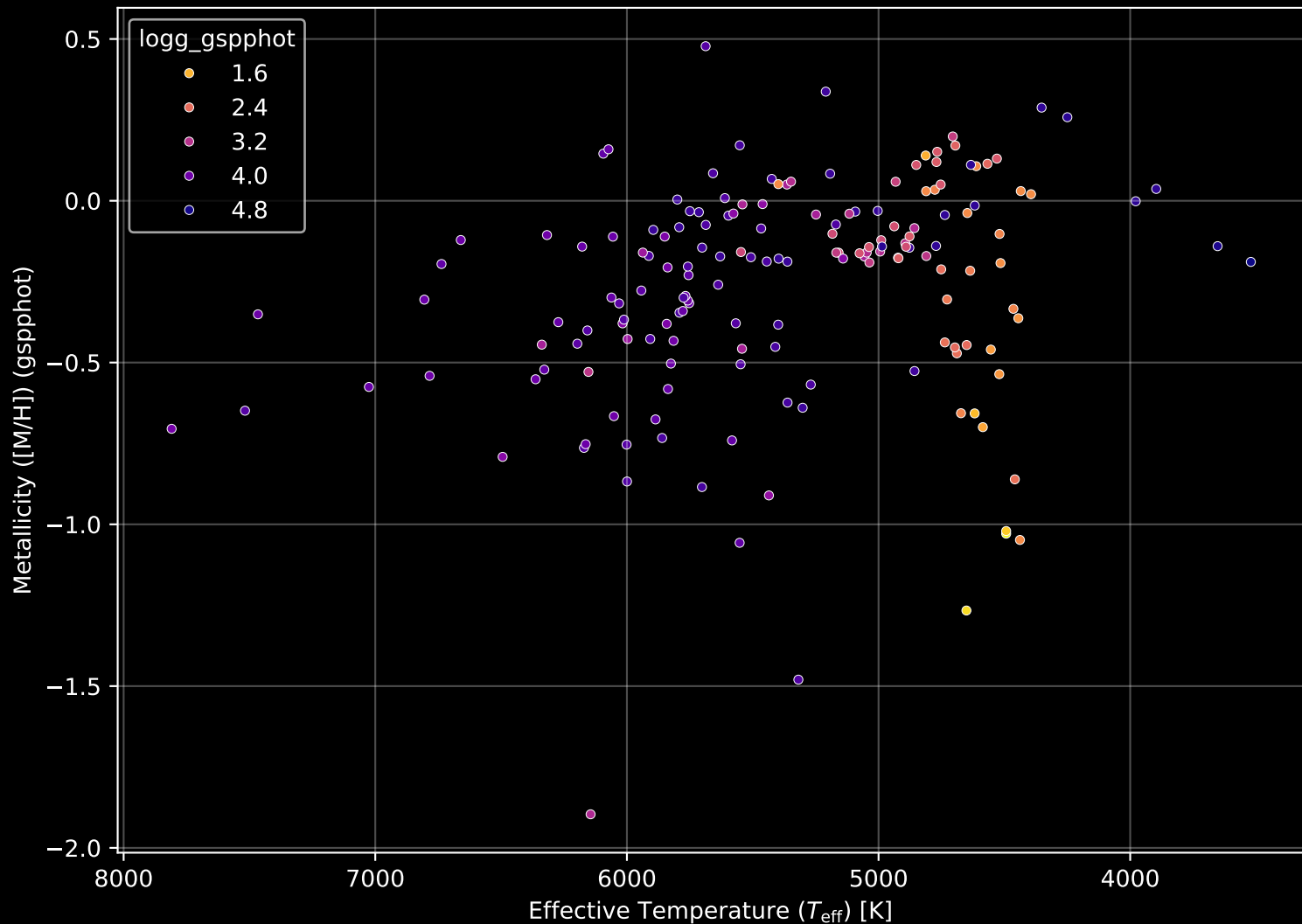
APOGEE DR17 Field: [283-23-O_TESS] Stellar Population Parameters (n= 168)
