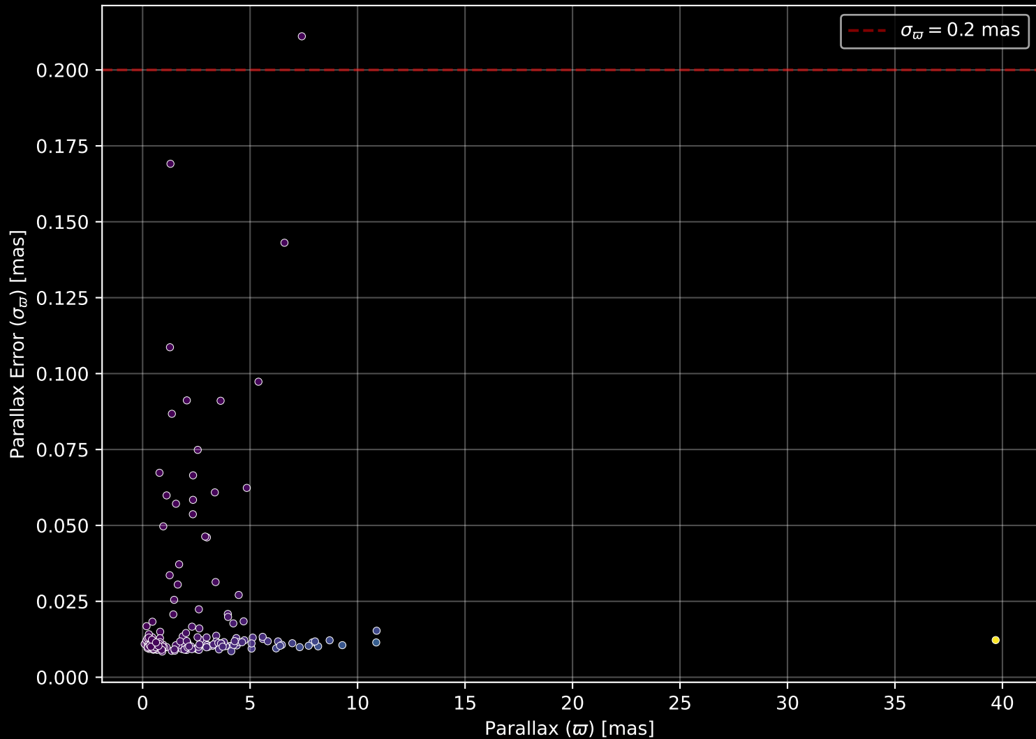
APOGEE DR17 Field: [283-23-O_TESS] Parallax Quality (n= 168)
