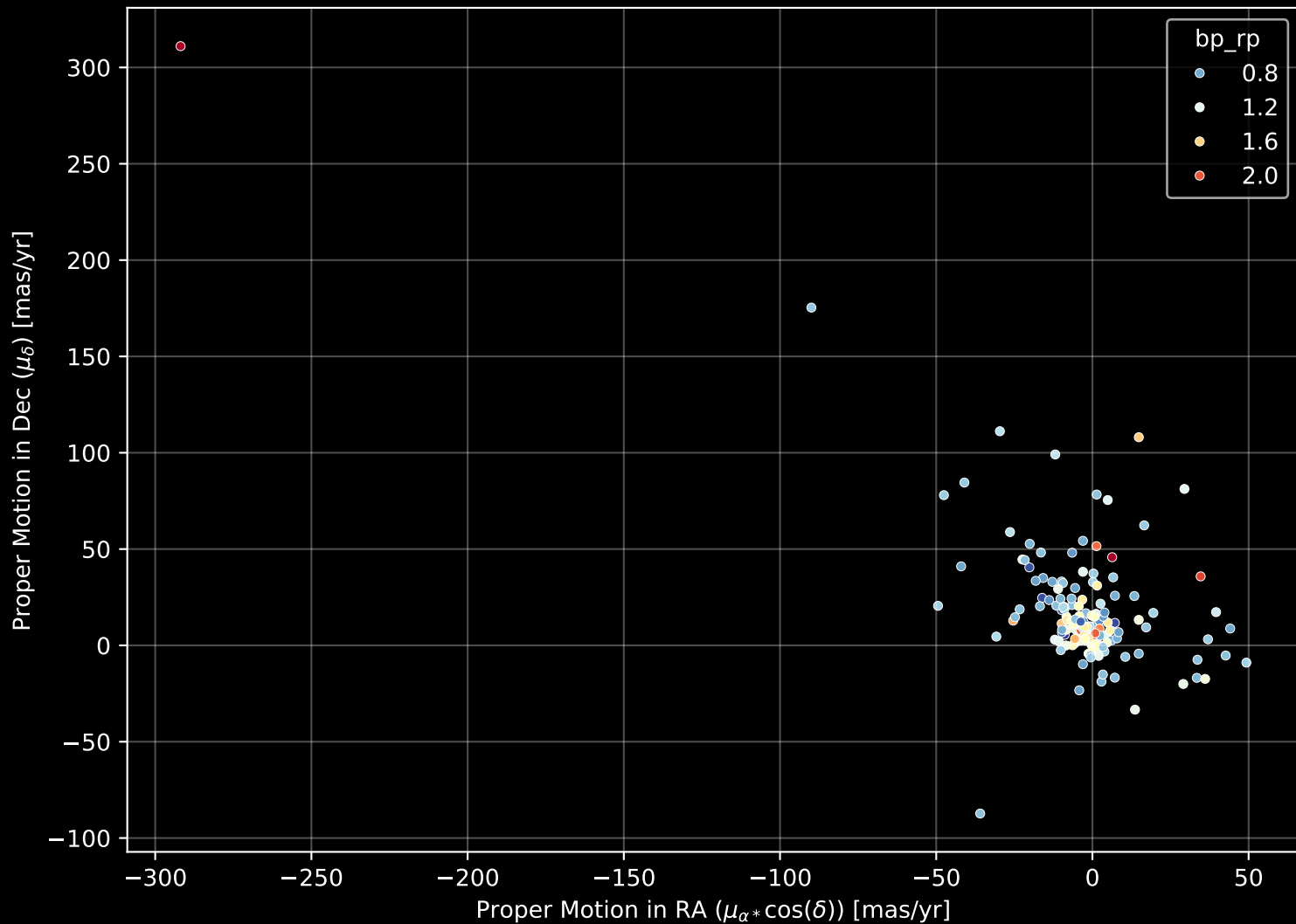
APOGEE DR17 Field: [283-23-O_TESS] Proper Motion Diagram (n= 168)
