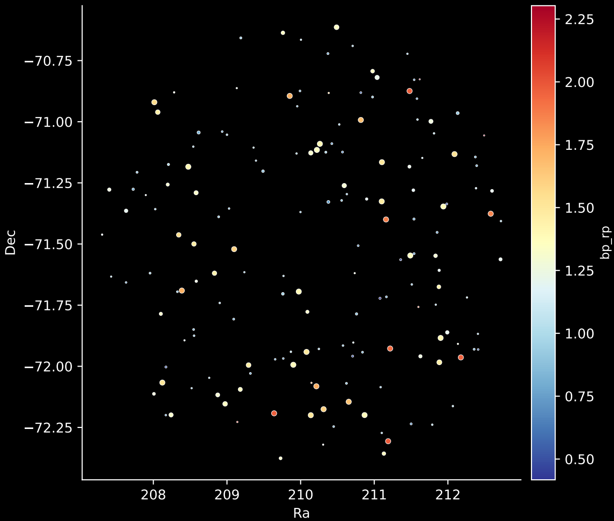
APOGEE DR17 Field: [283-23-O_TESS] Stars: 168
